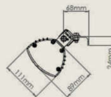
Zijaanzicht
