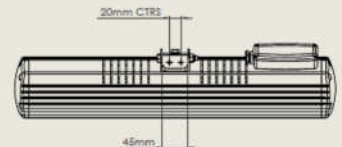
Achteraanzicht
