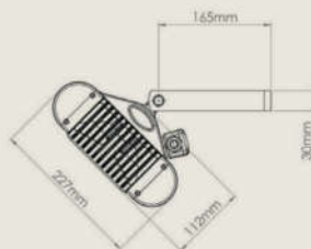
Zijaanzicht
