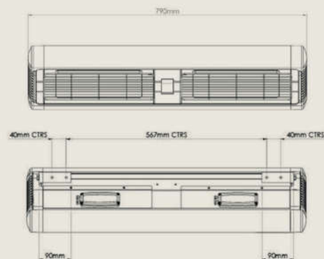
Achteraanzicht
