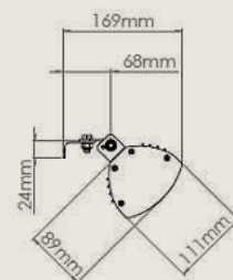
Zijaanzicht
