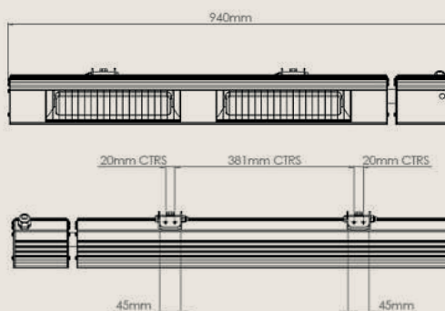
Achteraanzicht
