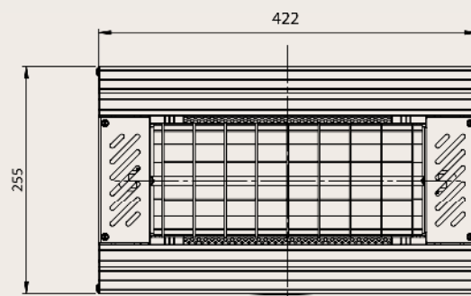
Vooraanzicht
